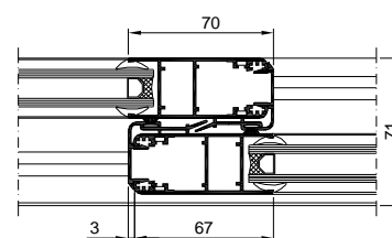
8 Parteluces
