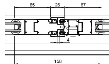
6 Marco Fijo
