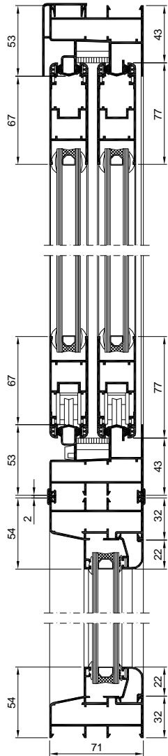
Sección 1 - 1
