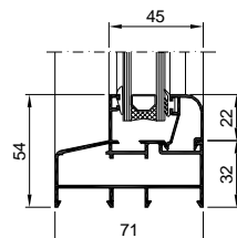
7 Marco Fijo
