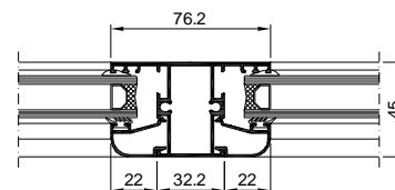
8 Parteluces
