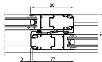
4 Cierre Central
